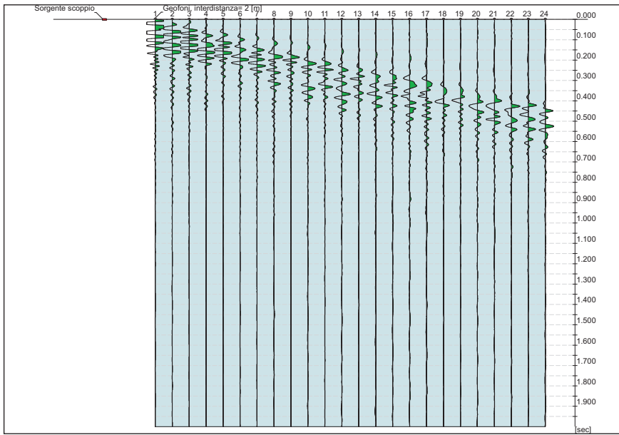
SISMOGRAMMA
