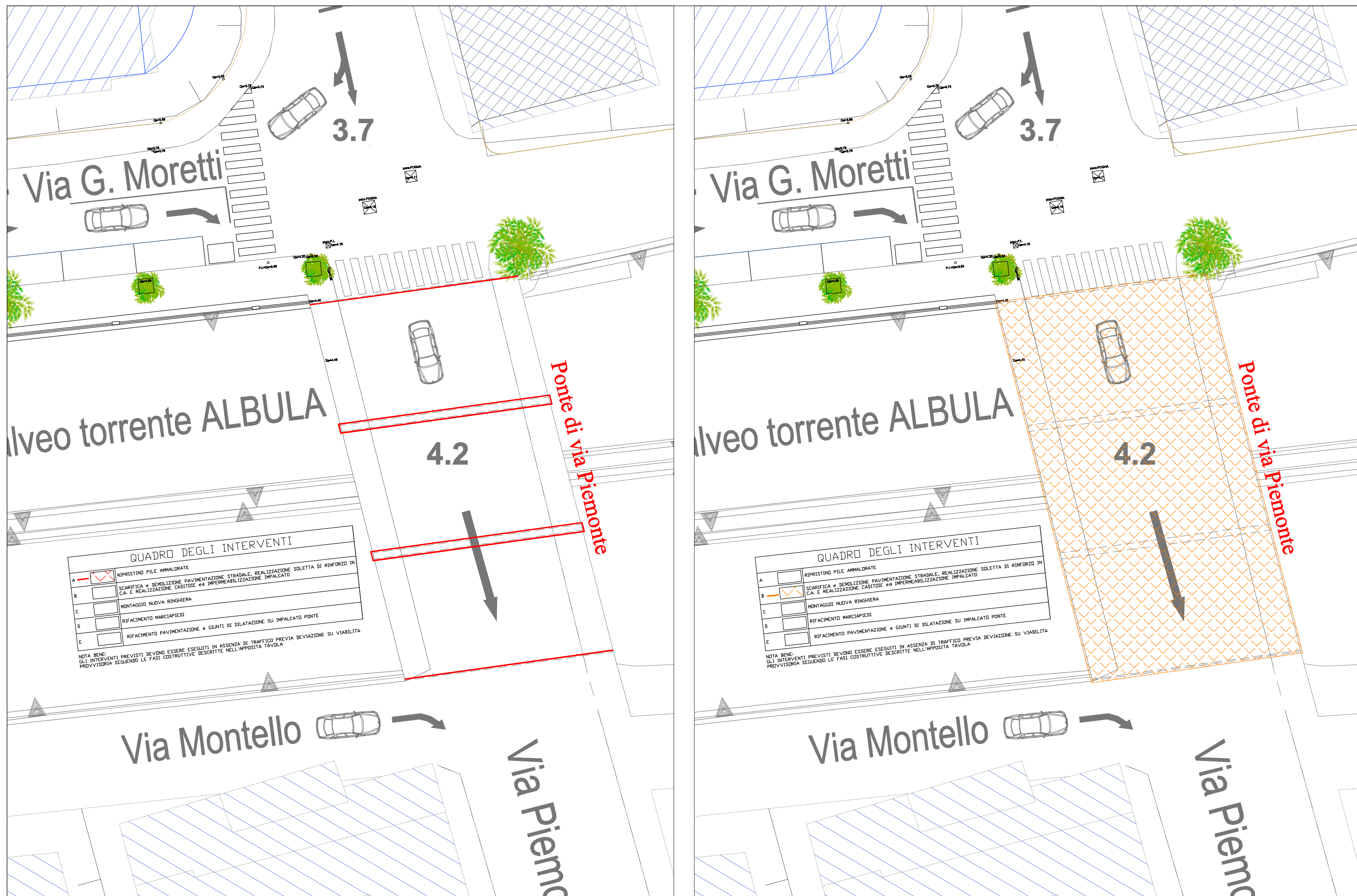
PLANIMETRIE con QUADRO degli INTERVENTI scala 1:200
