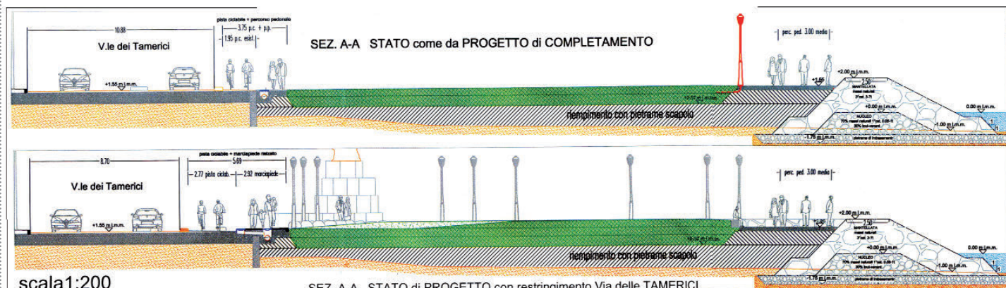
SEZ. A-A STATO di PROGETTO con restringimento Via delle TAMERICI
